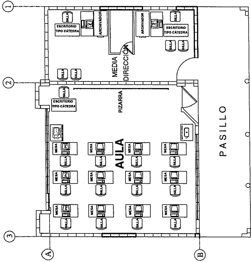
PLANTA DE MOBILIARIO MÓDULO DE UN AULA + MEDIA DIRECCIÓN
